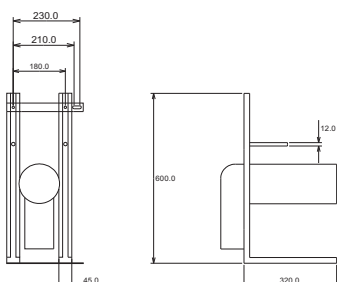
Art. 83B Attacco di fissaggio per WC e bidet sospesi con regolazione interasse fori da 180/230 € 15,00 netto (pezzo singolo) € 36,00 la coppia (WC + bidet sospeso)
