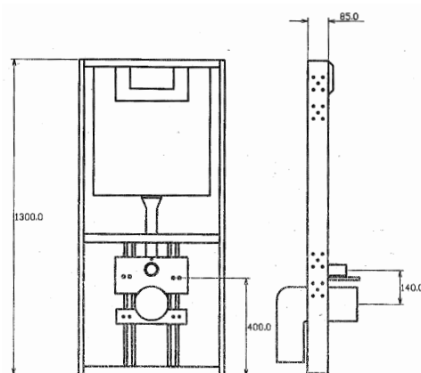
Art. 83/P2 Struttura metallica per fissaggio WC sospesi su pareti in cartongesso o cemento - completa di cassetta di scarico incasso doppio flusso € 156,00 netto (placca bianca) € 170,00 netto (placca cromo)
